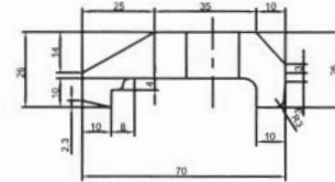
RAIL CLIP 30,37kg 상판
