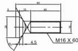
M16 BOLT
