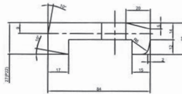
RAIL CLIP 50Kg 상판 ①
