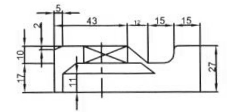
RAIL CLIP 73Kg 하판 ②
