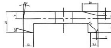
RAIL CLIP 73Kg 상판 ①
